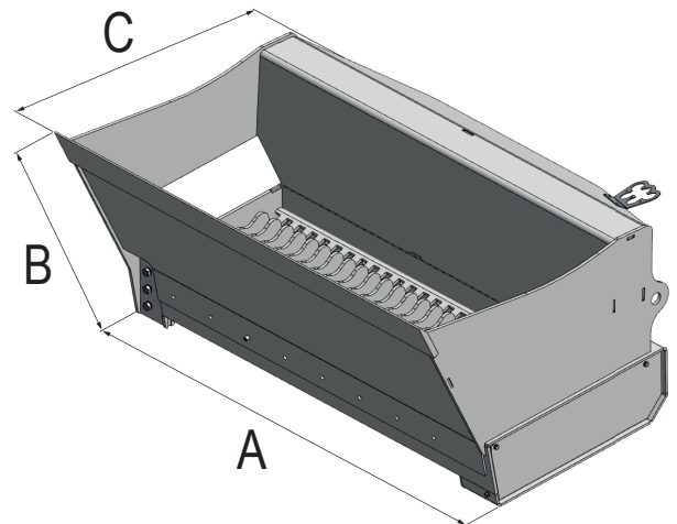
Габариты (мм)
